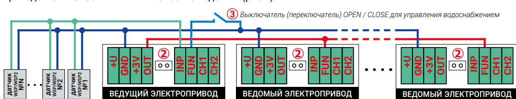
Рис. 1. Объединение в систему нескольких шаровых электроприводов из серий GIDROLOCK WINNER
