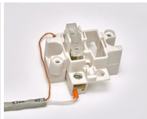
Фото 22. Подключение проводного выключателя
