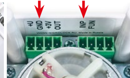
Фото 13. Клеммы подключения проводных датчиков — INP, GND
