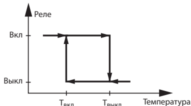
Рис. 10. Гистерезис работы.
