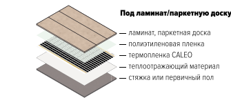
Рис. Схема монтажа теплого пола CALEO под ламинат или паркетную доску
