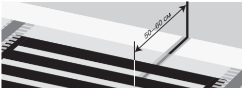
Рис. 4. Схема установки датчика температуры пола
