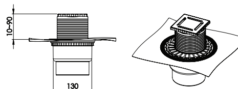
Вертикальный сифон D50/75/110 - H120 мм
