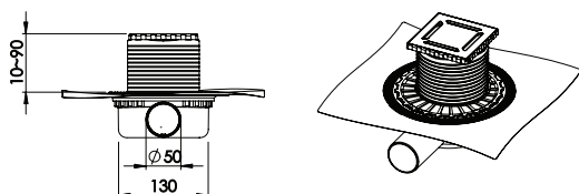
Боковой S-образный сифон D50-H65 мм
