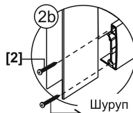
Шуруп ST4x35
