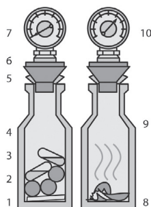
Рис. 10. Прибор СМ (измерение при помощи карбидно-кальциевого метода)
