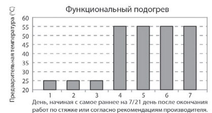
Рис. 15. Функциональный подогрев
