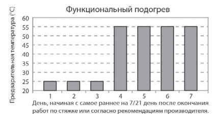
Рис. 15. Функциональный подогрев
