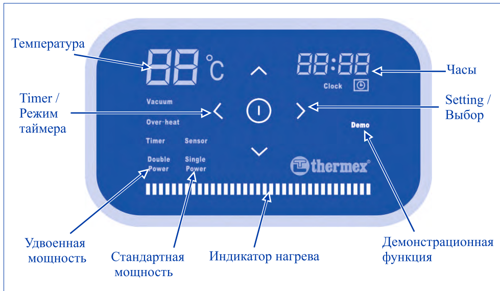
Рис. 6. Электронная панель управления (вариант 2)
